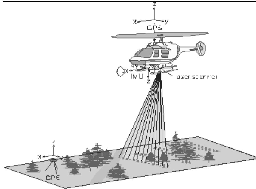
FIGURE 3 Composantes d'un système LIDAR (d'après Lillesand et Kiefer 2000)
